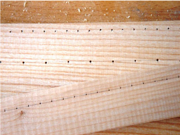
Anzeichnen und Vorstechen der Bohrlöcher
